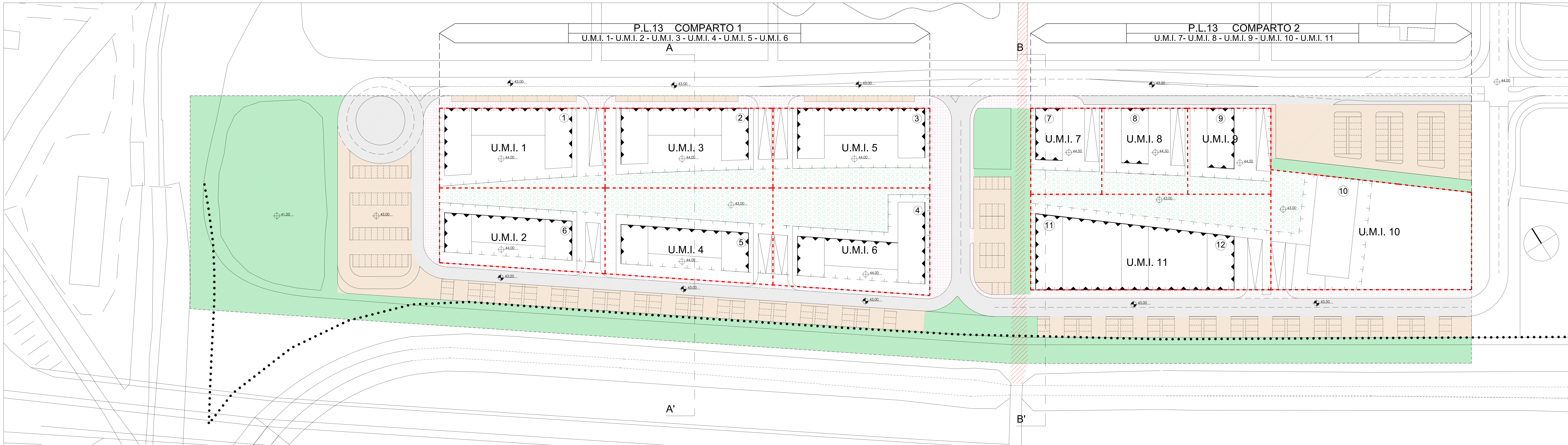
PLANIMETRIA USO DEL SUOLO
